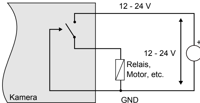
Abb. 6: Anschluss der digitalen Ausgänge (PLCOUT/TriggerOUT)
