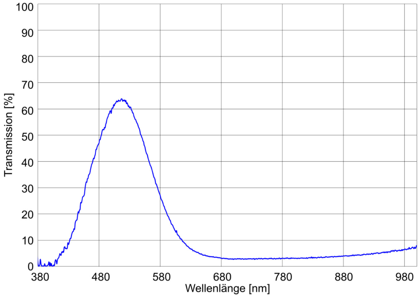
Transmission Farbfilter Grün G06
