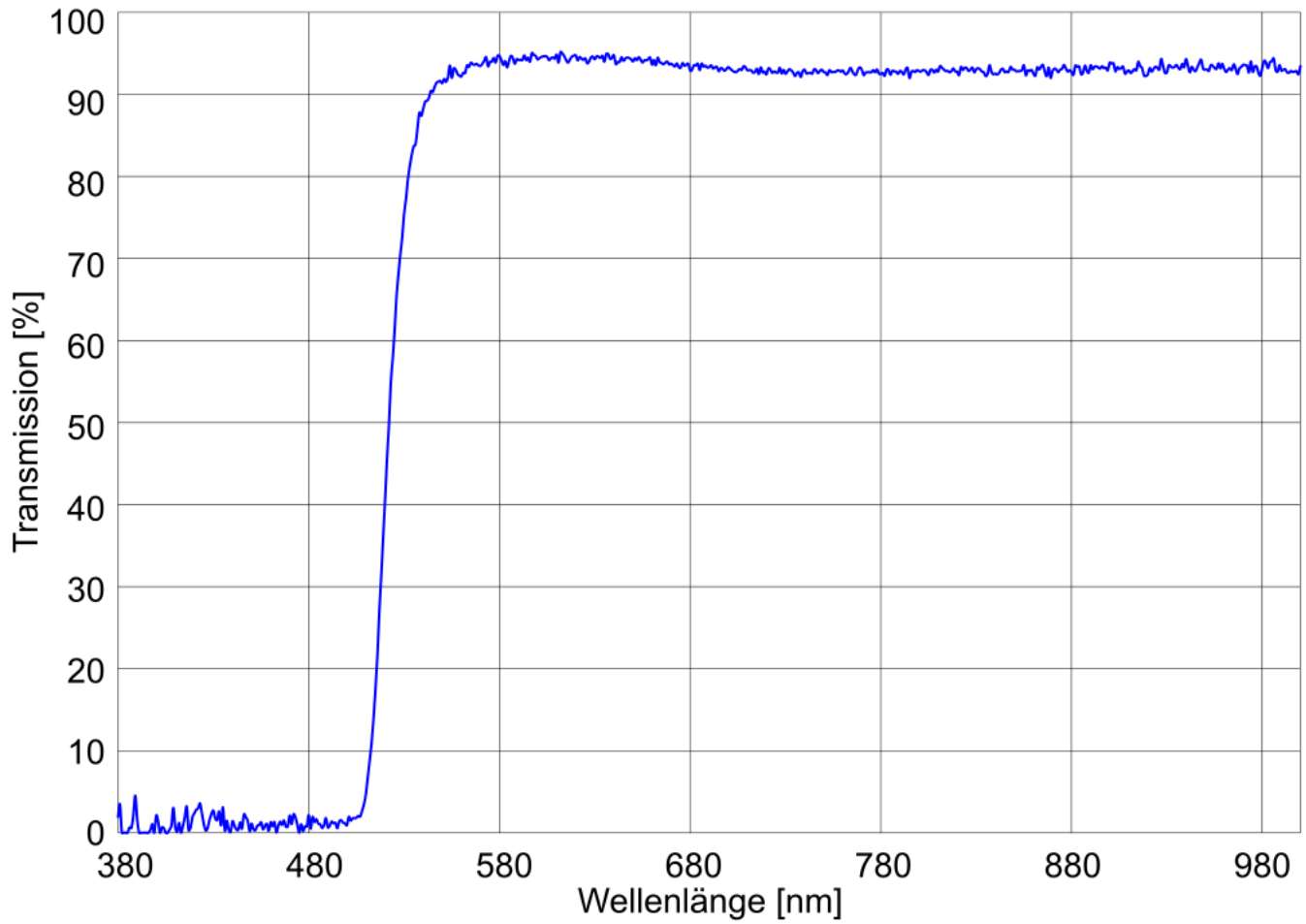
Transmission Farbfilter Gelb OG530
