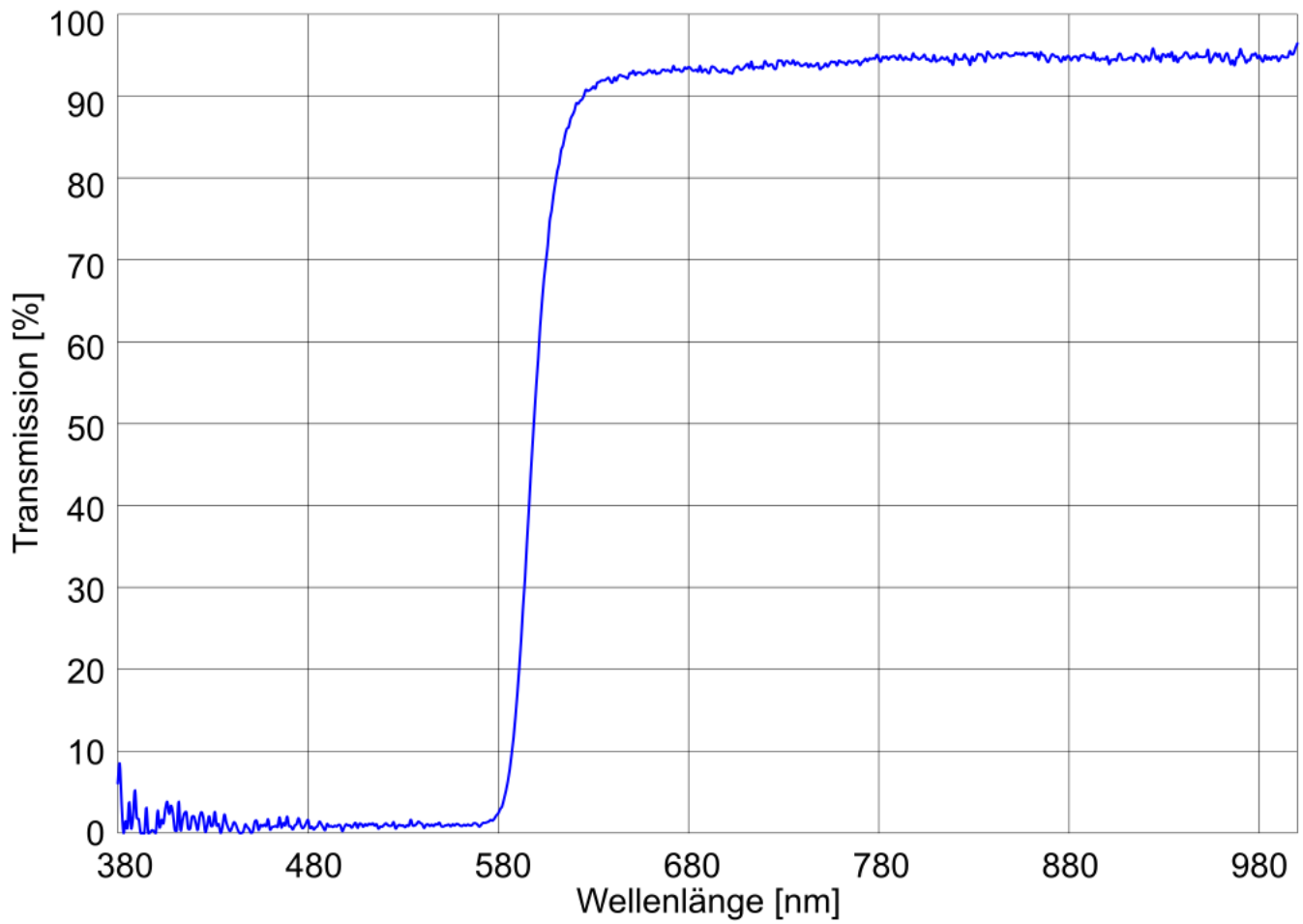
Transmission Farbfilter Rot RG610
