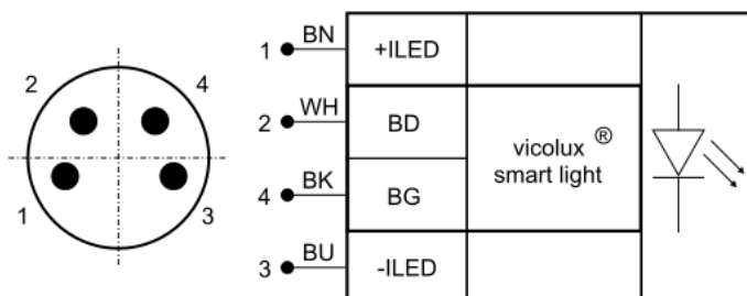
Anschlussbelegung: M8-Stecker
