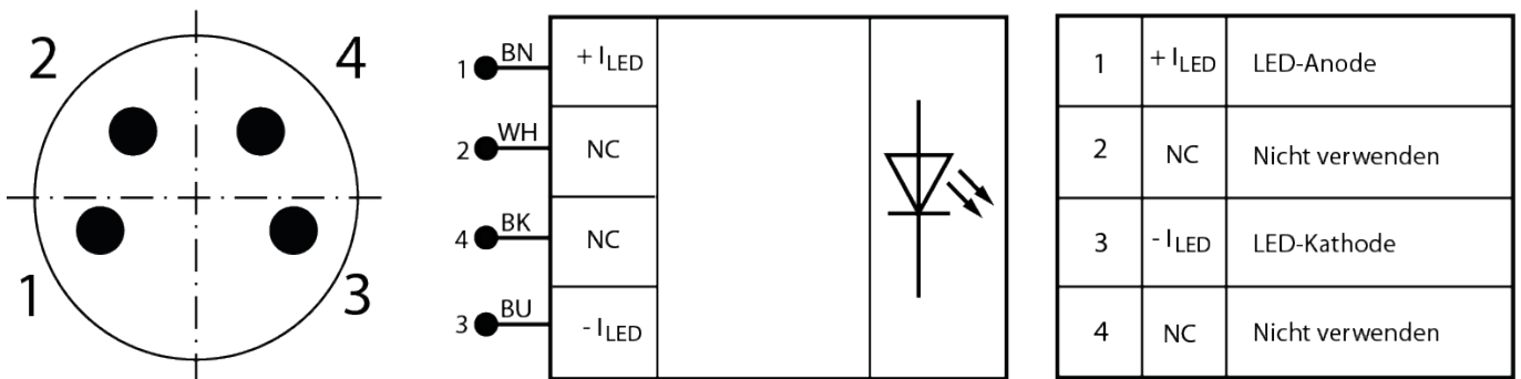
Anschlussbelegung M8-Stecker
