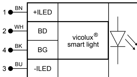
Abb. 8: Anschlussschema vicolux smart light
