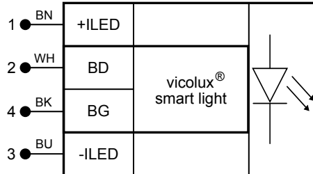
Abb. 9: Anschlussschema vicolux smart light
