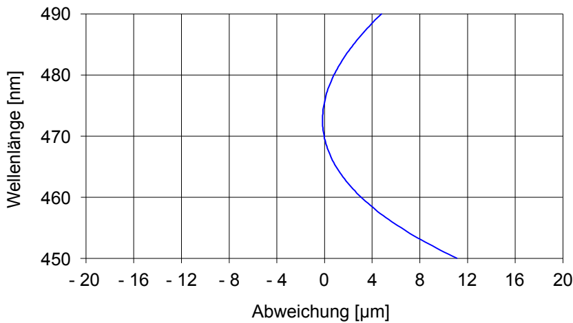
Abb. 7: Farblängsfehler – wellenlängenabhängig
