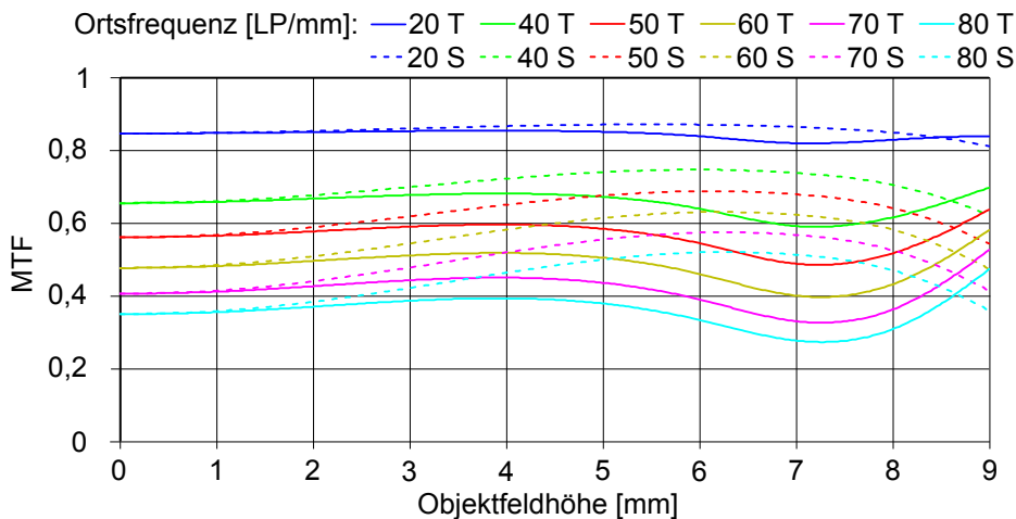
Abb. 5: MTF - bildfeldabhängig (470 nm, F10)
