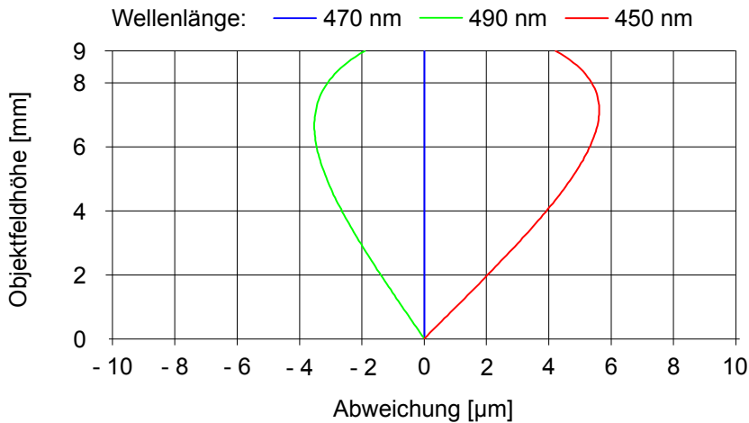
Abb. 6: Farbquerfehler – wellenlängenabhängig
