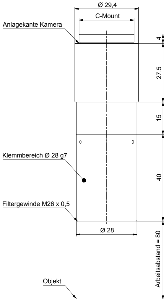
Abb. 10: Technische Zeichnung
