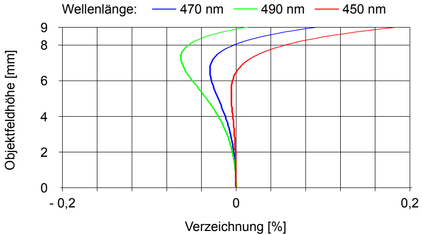
Abb. 8: Verzeichnung – wellenlängenabhängig
