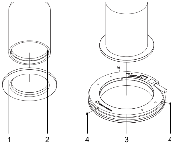
Abbildung 5: Montage mittels Adapterring (allgemeine Darstellung)
