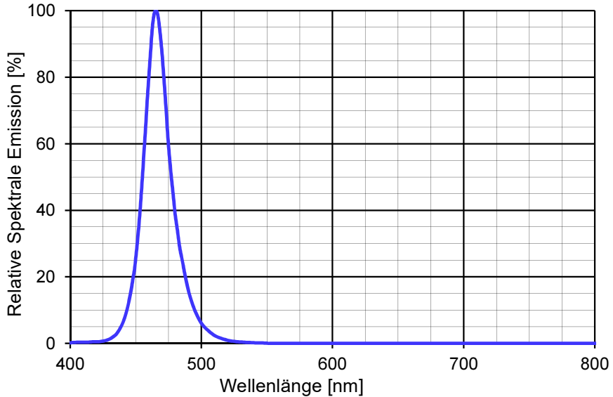
Abbildung 9: Spektrale Emission
