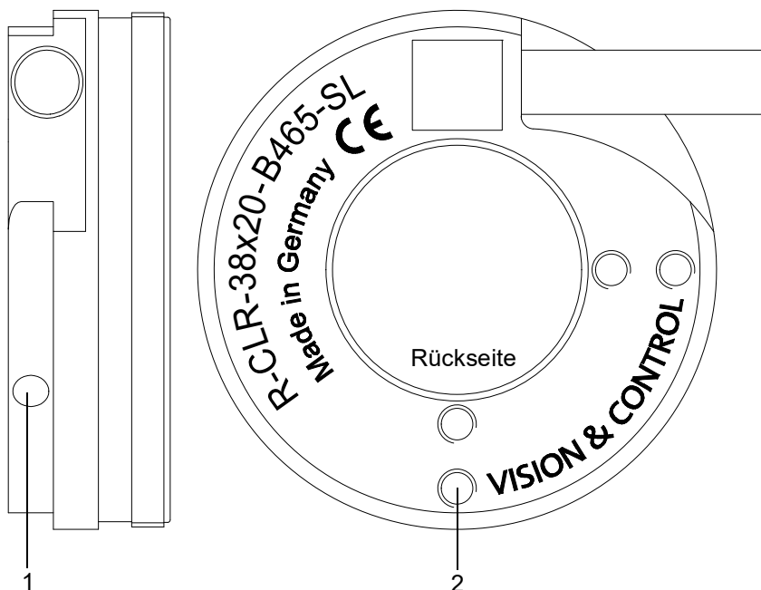
Abbildung 4: Position der Montagebohrungen und Gewindestifte
