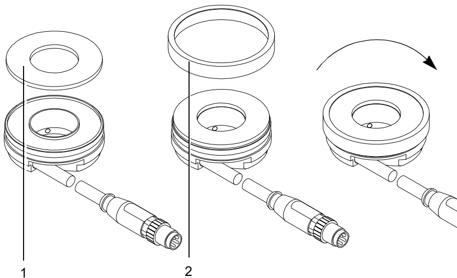
Abbildung 6: Optisches Zubehör montieren
