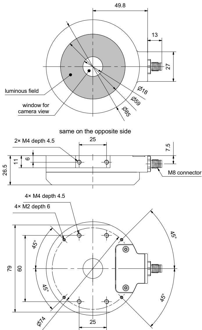
Abbildung 3: Maßzeichnung (alle Maßangaben in mm)
