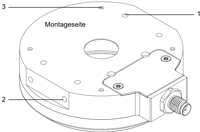
Abbildung 4: Montagebohrungen
