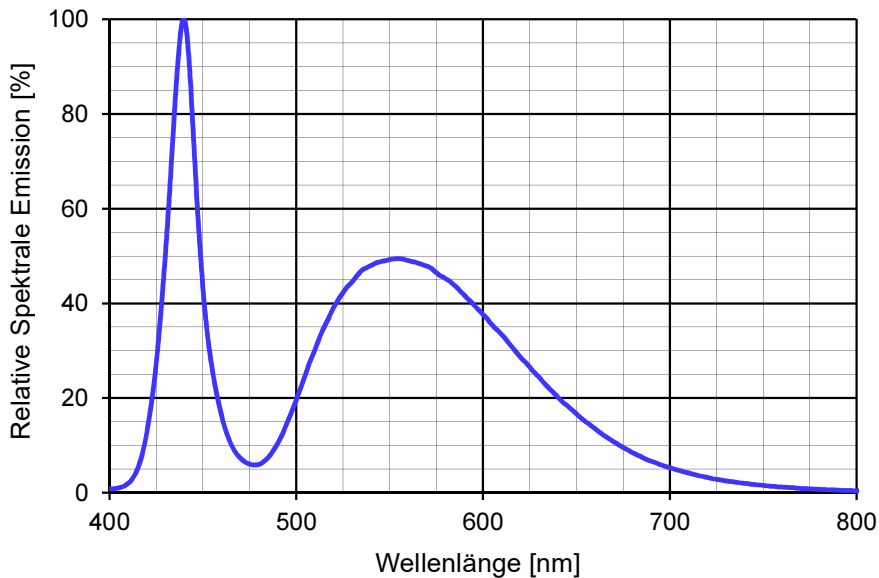
Abbildung 7: Spektrale Emission
