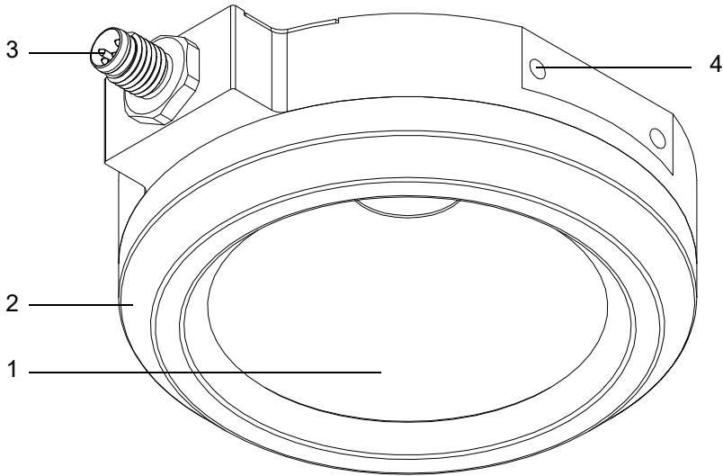
Abbildung 2: Geräteaufbau
