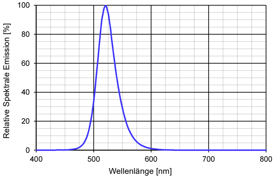
Abbildung 7: Spektrale Emission
