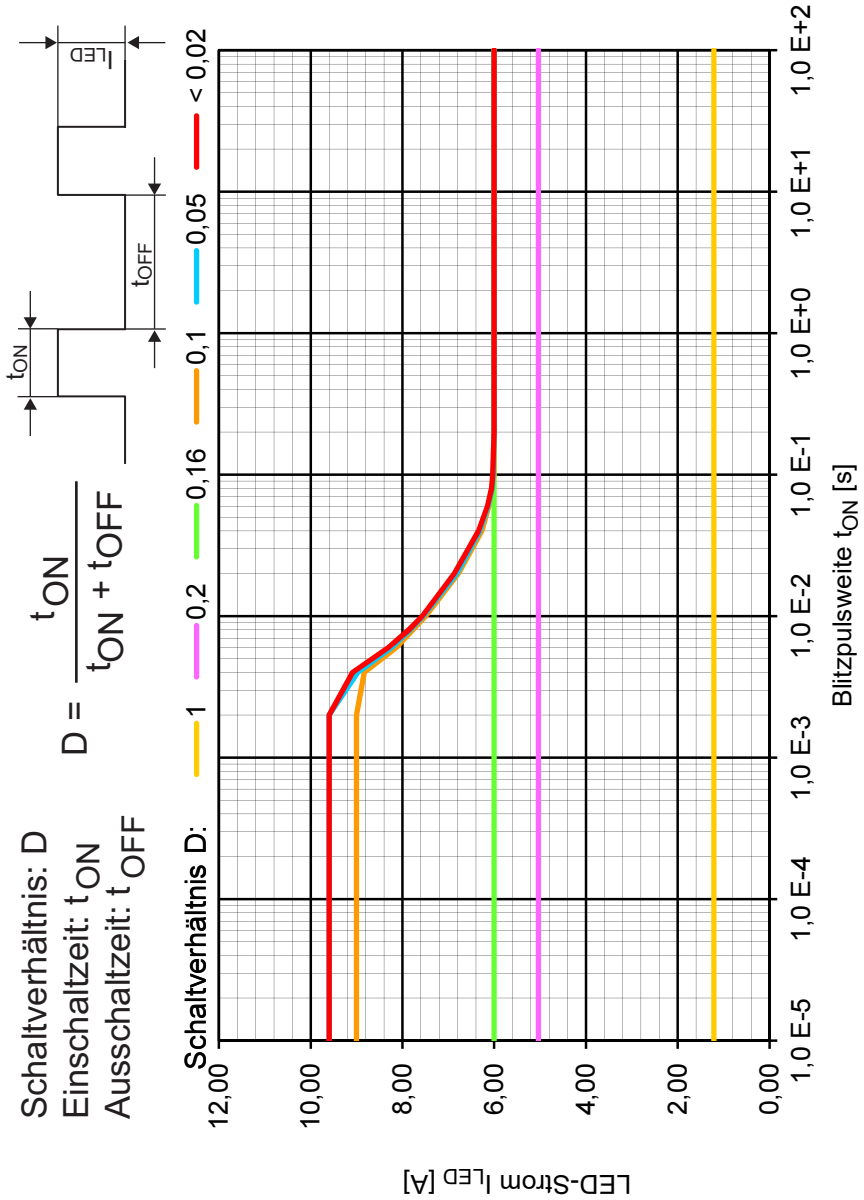
Abbildung 6: Impulsbelastung bei Umgebungstemperatur = 25 °C
